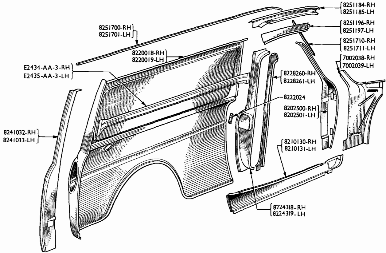
BODY SIDE - VAN
