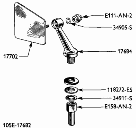
105E-17682
