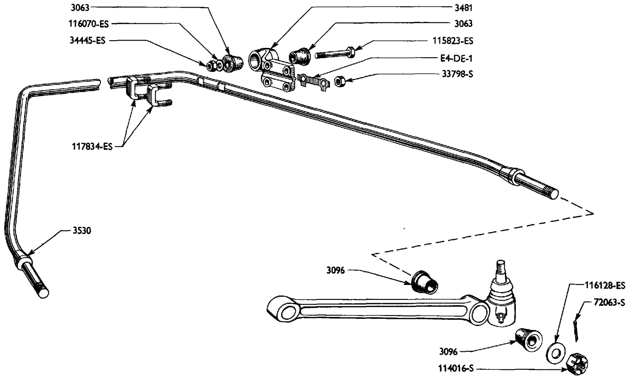
STABILIZER BAR
