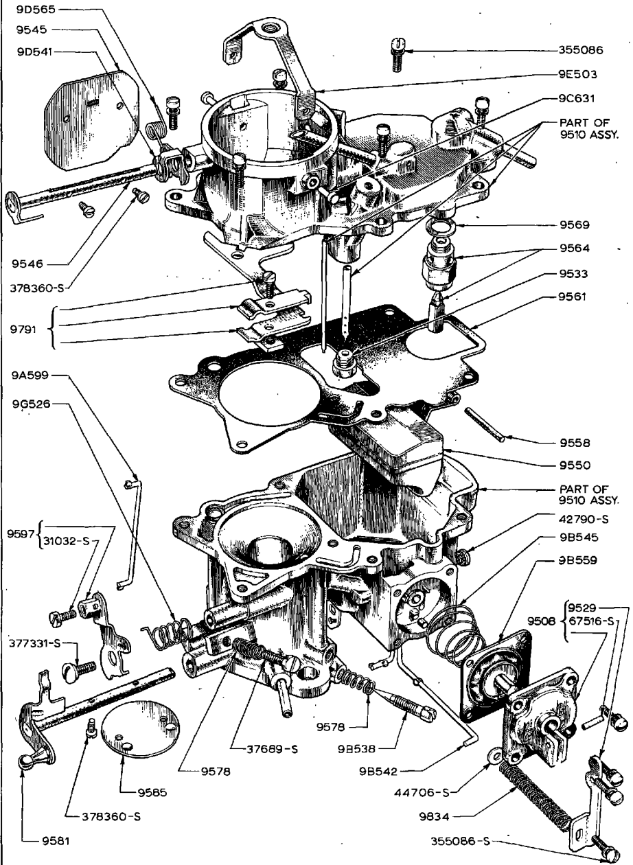
CARBURETTOR - 997 C.C.
