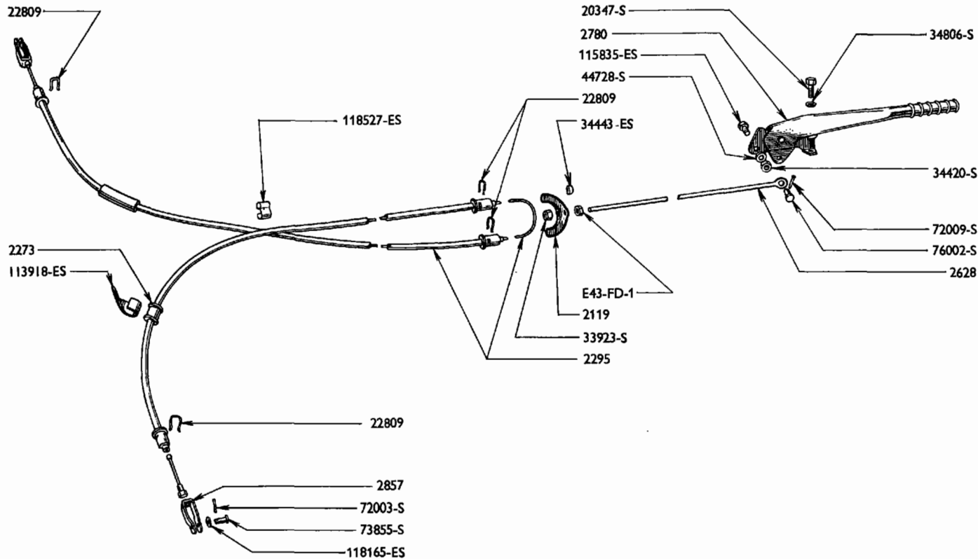
HANDBRAKE-VAN
