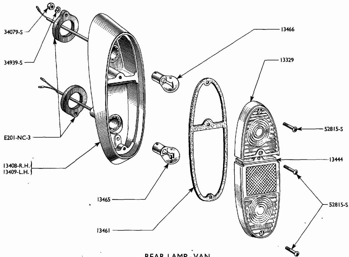
REAR LAMP - VAN
