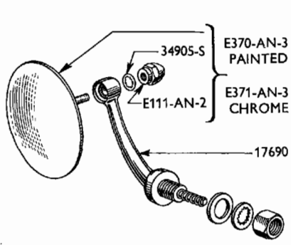
VAN DOOR FITTING
